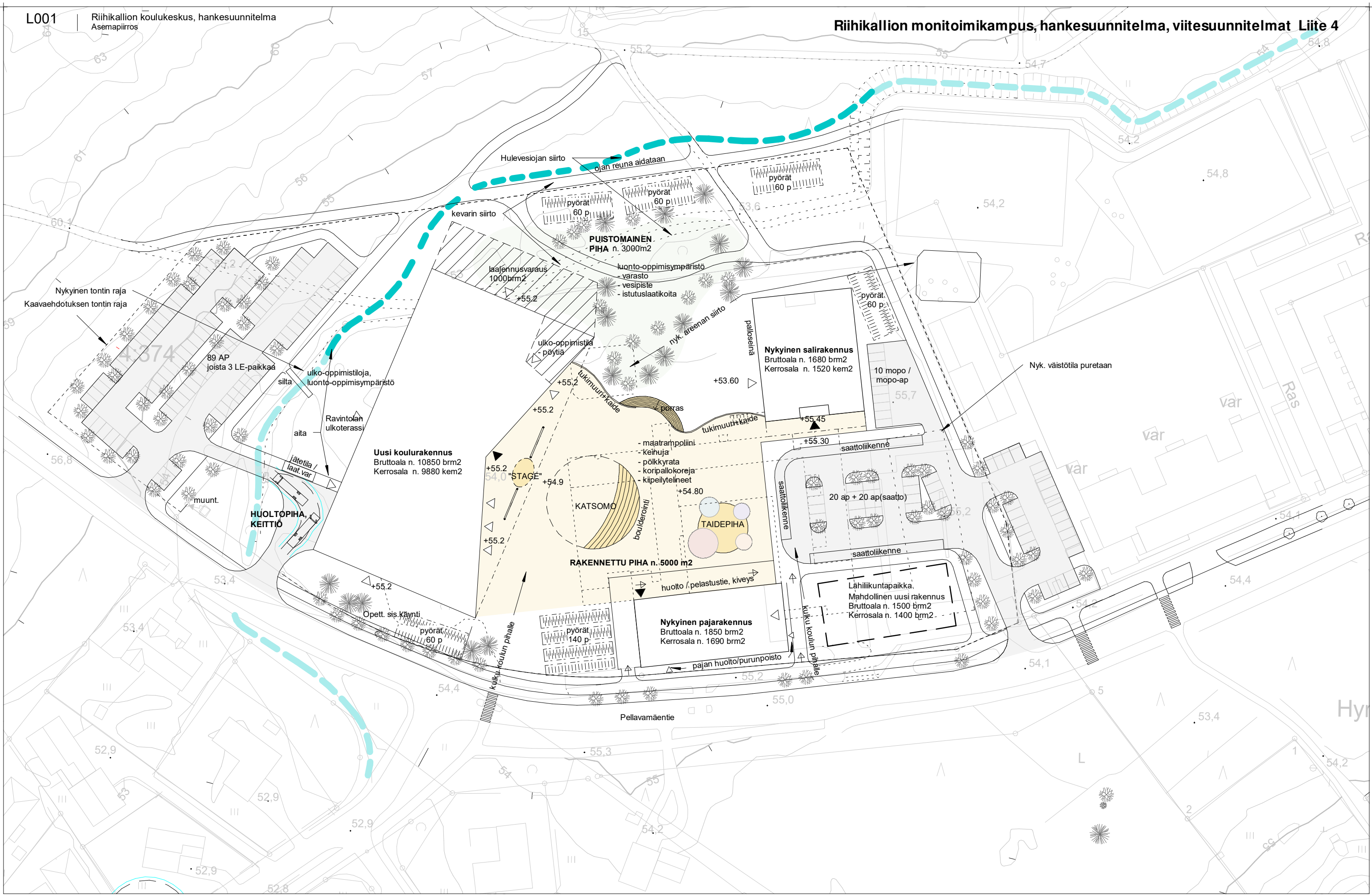
LUONNOS asemapiirros 1 : 1000
