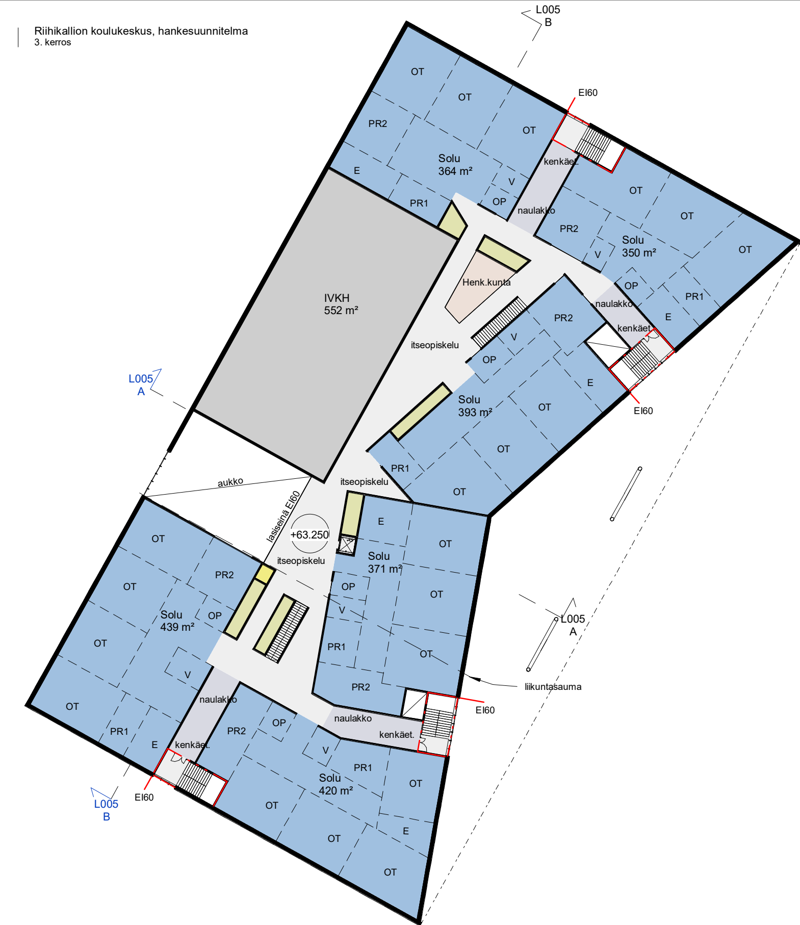
LUONNOS 3. kerros 1 : 450
