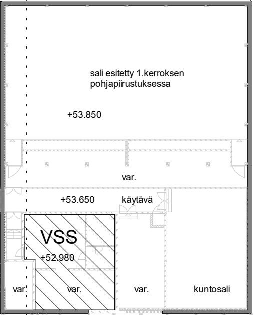
LUONNOS 0. kerros 1 : 450
