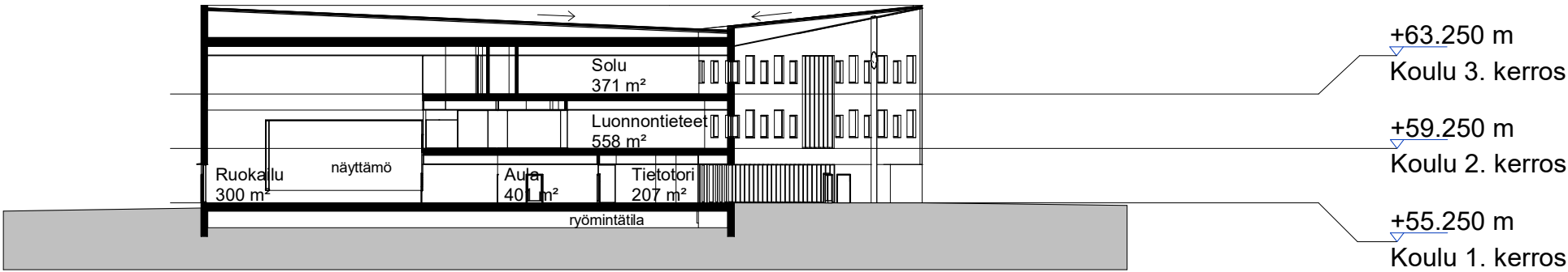
Leikkaus A 1 : 450
