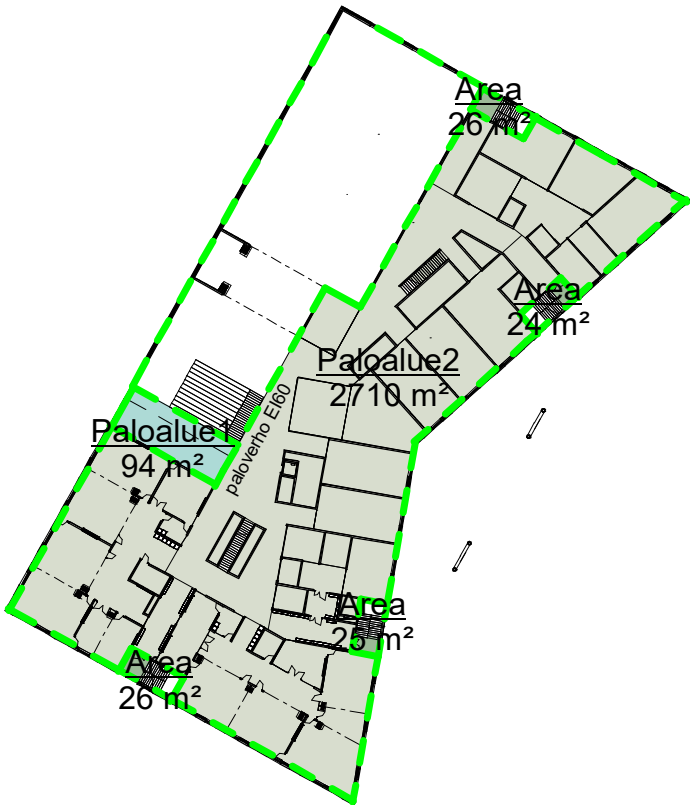
Koulu 2. kerros 1 : 1000
