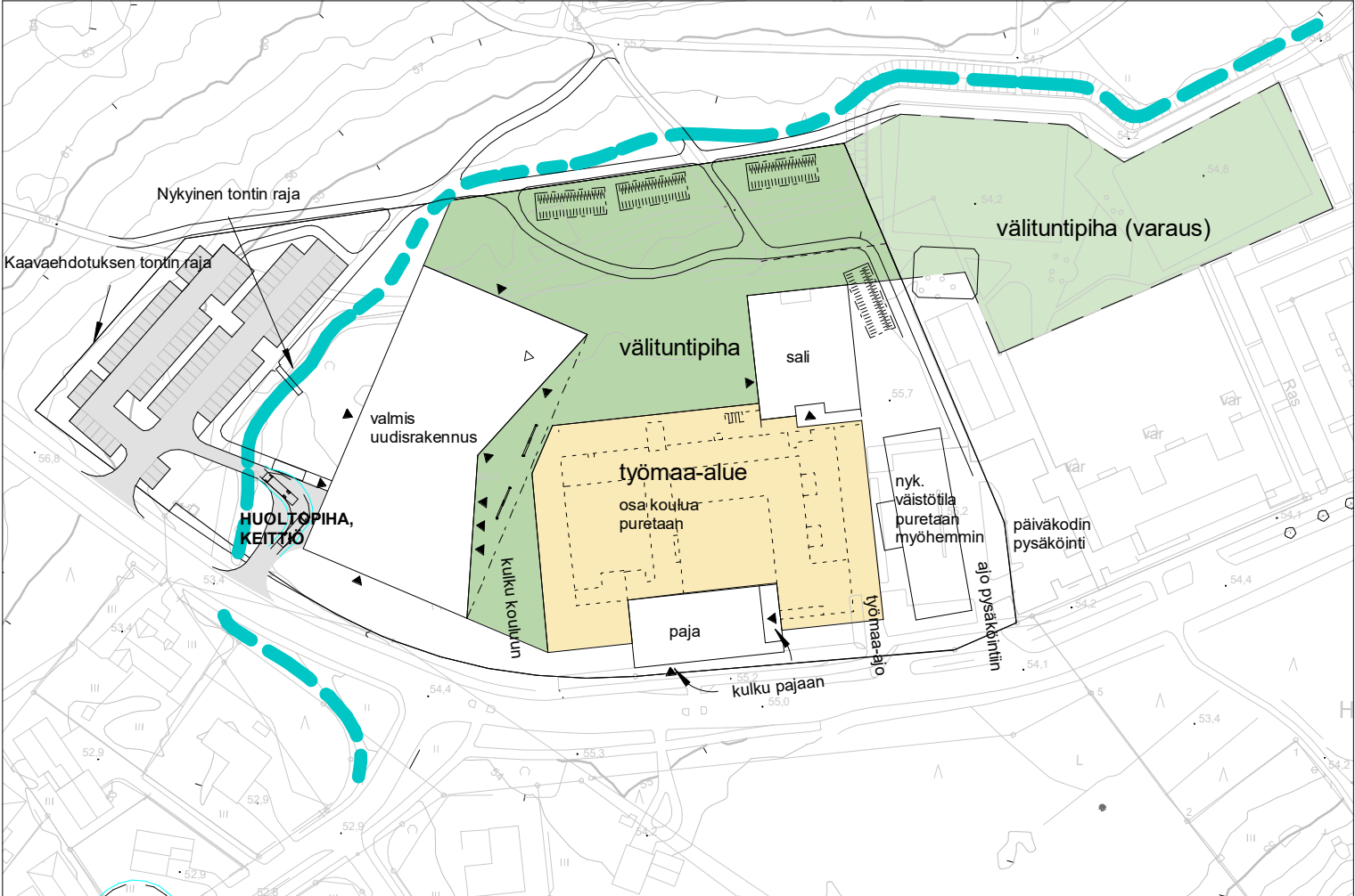
LUONNOS asemapiirros PURKU 1 : 2000
