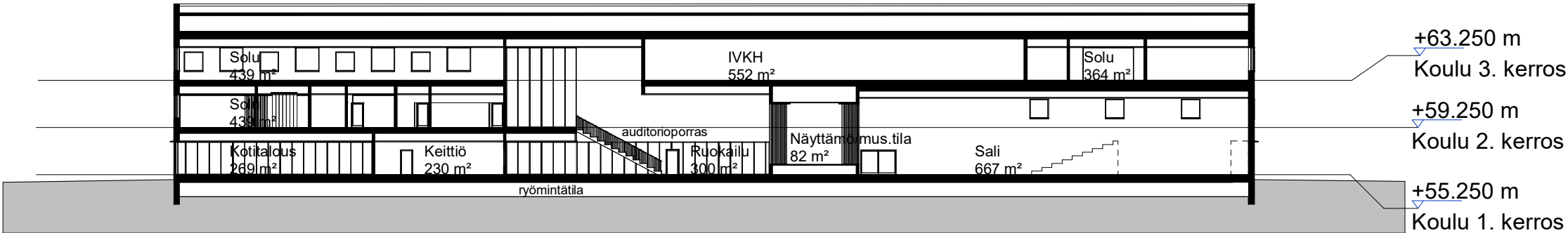
Leikkaus B 1 : 450
