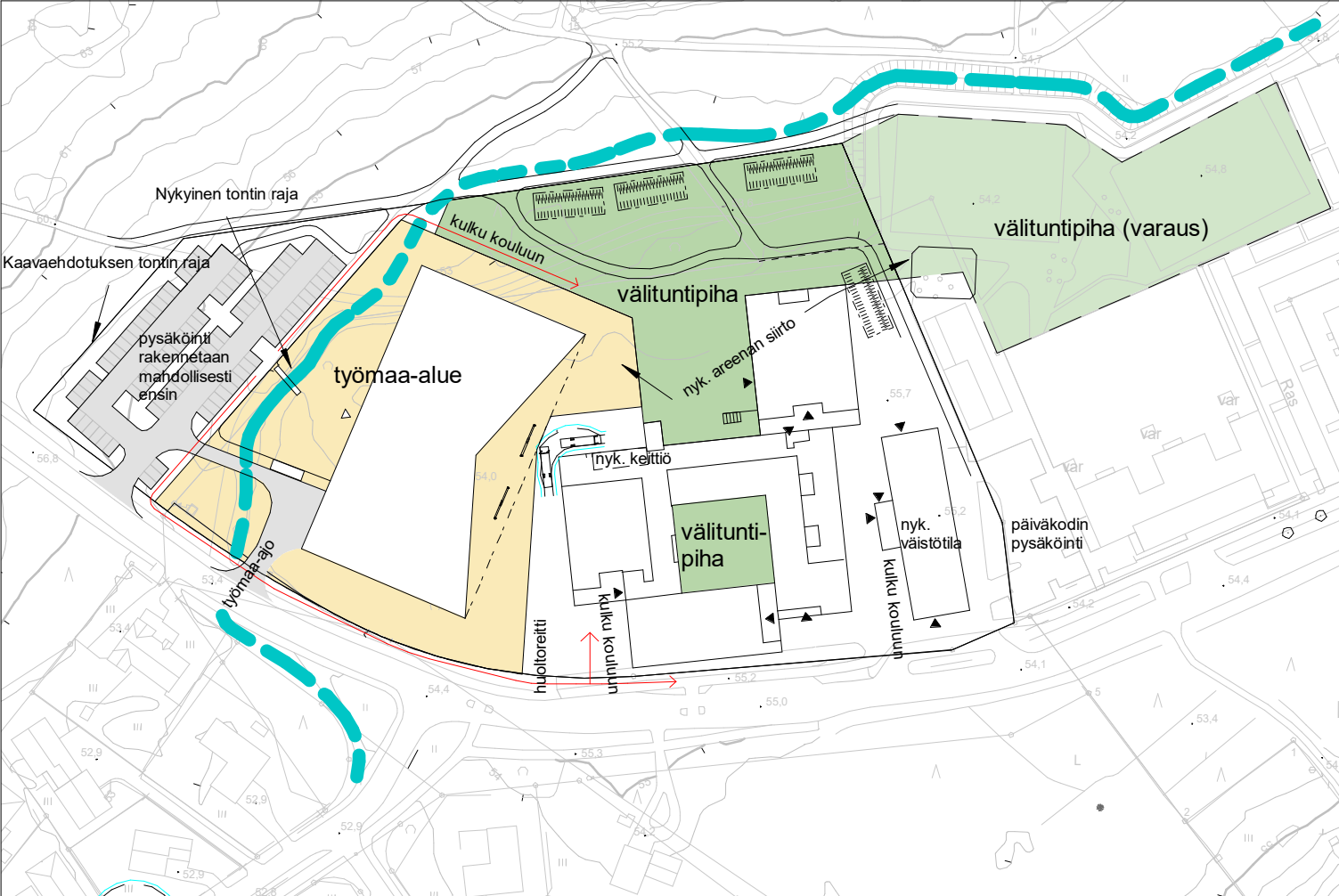
LUONNOS asemapiirros RAKENTAMINEN 1 : 2000
